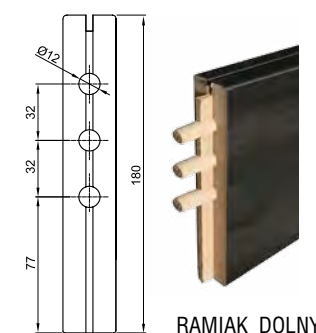
RAMIAK DOLNY
