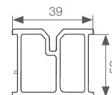
wymiary legara aluminiowego wysokiego (mm)
