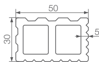
wymiary legara (mm)
