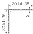
wymiary kątownika aluminiowego (mm)
