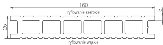
wymiary deski (mm)
