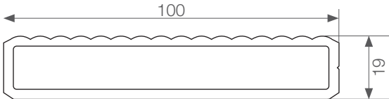
uniwersalny profil WPC
